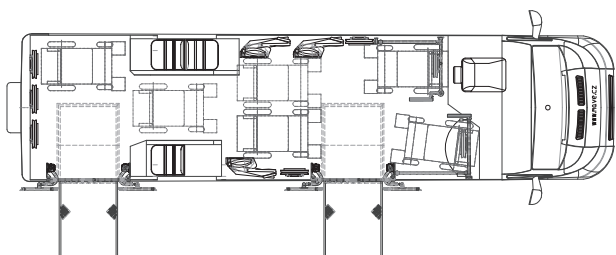
Dvounápravový autobus CiBus Ena Z Maxi - vozíčkáři
