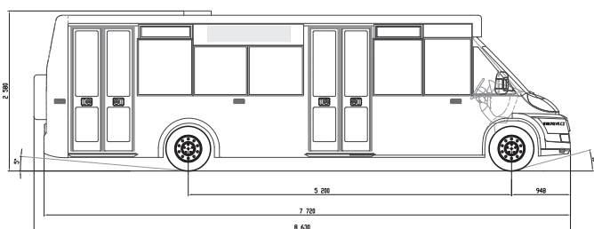
Dvounápravový autobus CiBus Ena Z
